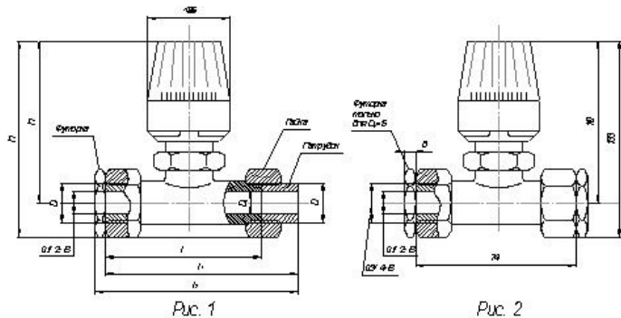
Терморегулятор прямой (варианты 1 и 2)
