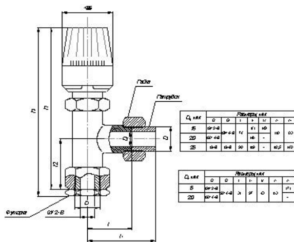
Терморегулятор угловой
